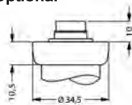
G1" DIN 3852
