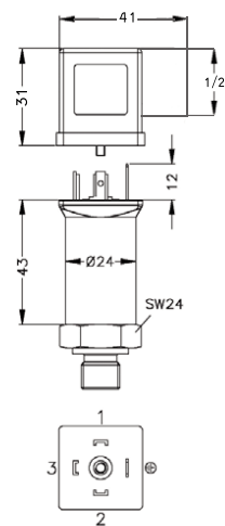
DIN 43650 A 1/2" NPTF conduit fitting
