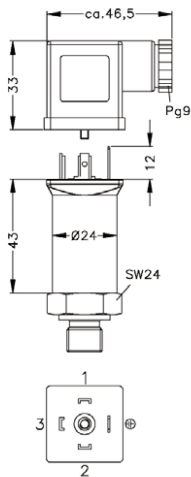
ISO 4400 (IP 65)
